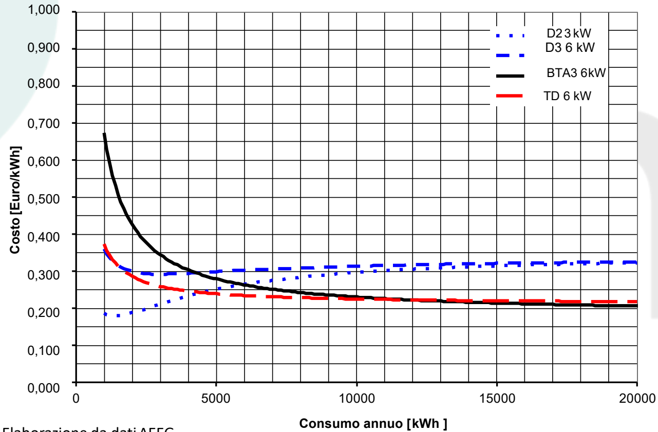
Costi medi energia elettrica in funzione di consumo e contratto (inclusa IVA 10%)
